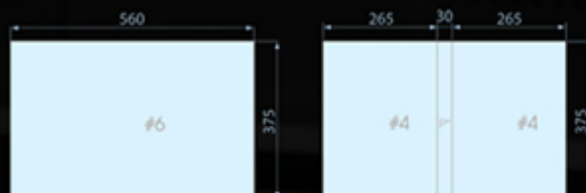
Wymiary wkładów (mm)
